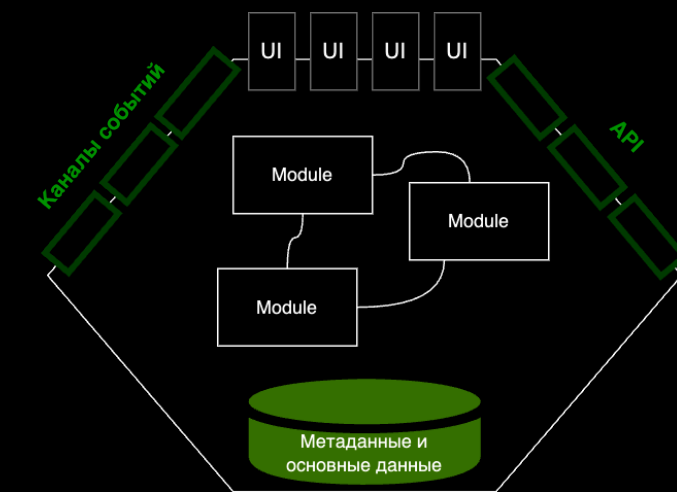
СБС данных
