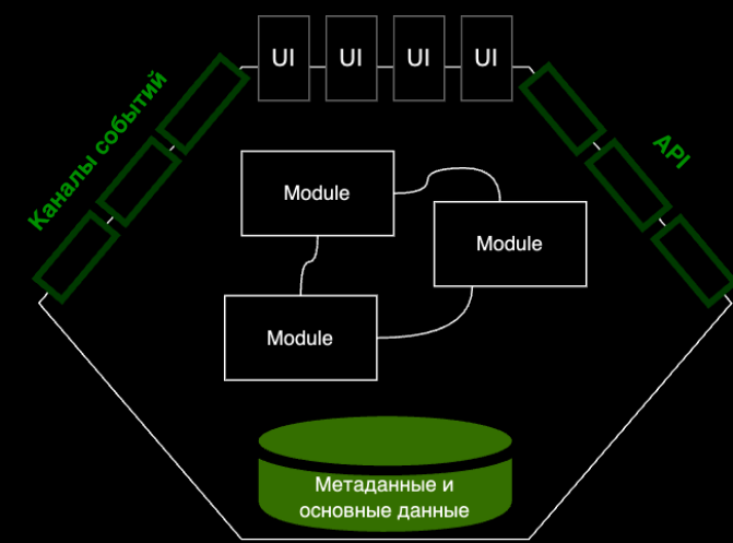
СБС сущности
