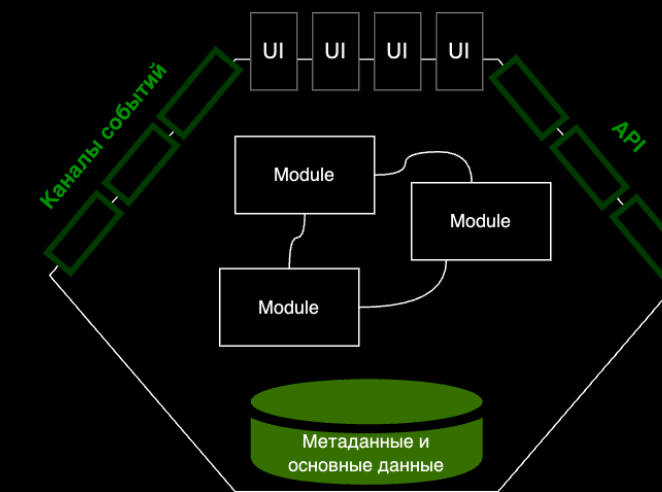
СБС аналитики
